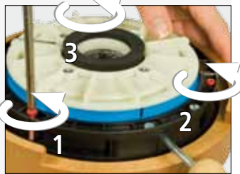
Bild 3 3 Transport- schrauben (rot markiert) entfernen.
